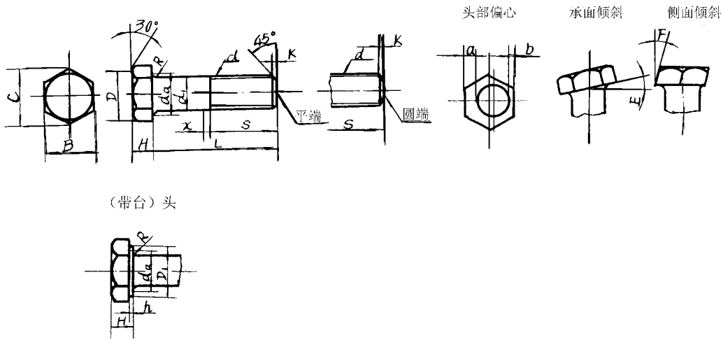
附表 1.1 六角头螺栓、精
