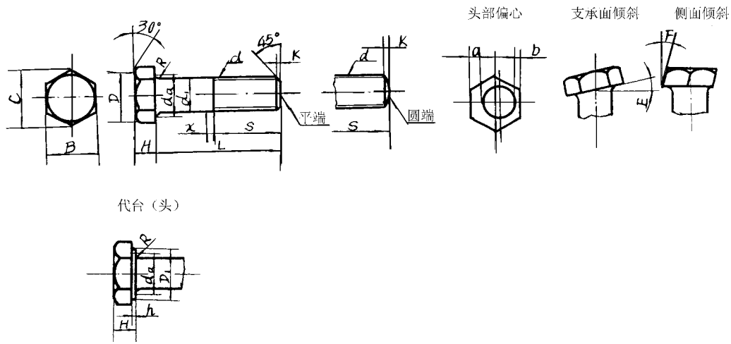
附表 2.2 小六角头螺栓、中
