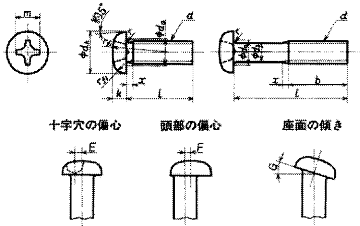
附属書付表 1 なべ小ねじの形状・寸法
