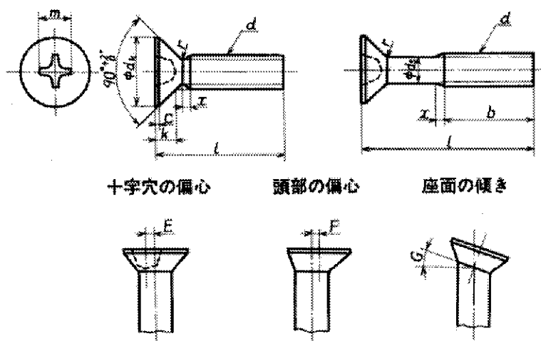
附属書付表 2 皿小ねじの形状・寸法
