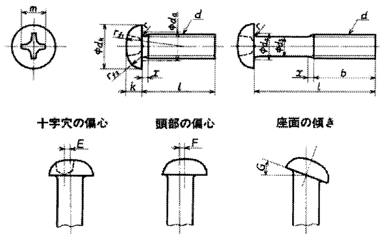
附属書付表 6 丸小ねじの形状・寸法
