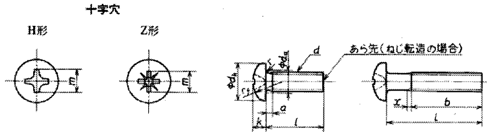
付表1 十字穴付きなべ小ねじの形状・寸法
