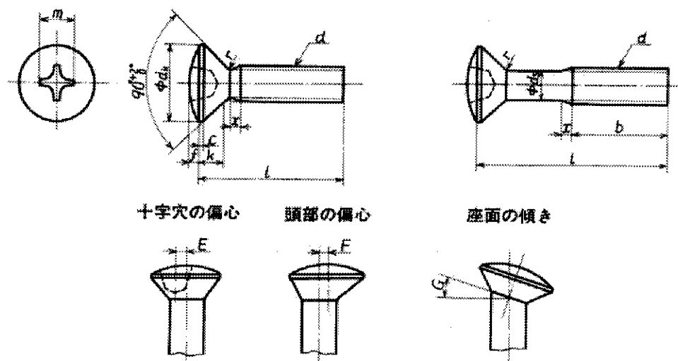
附属書付表 3 丸皿小ねじの形状・寸法
