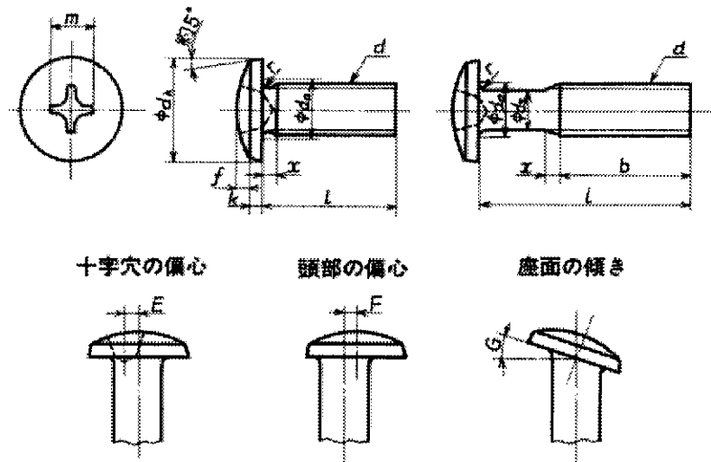
附属書付表 5 バインド小ねじの形状・寸法
